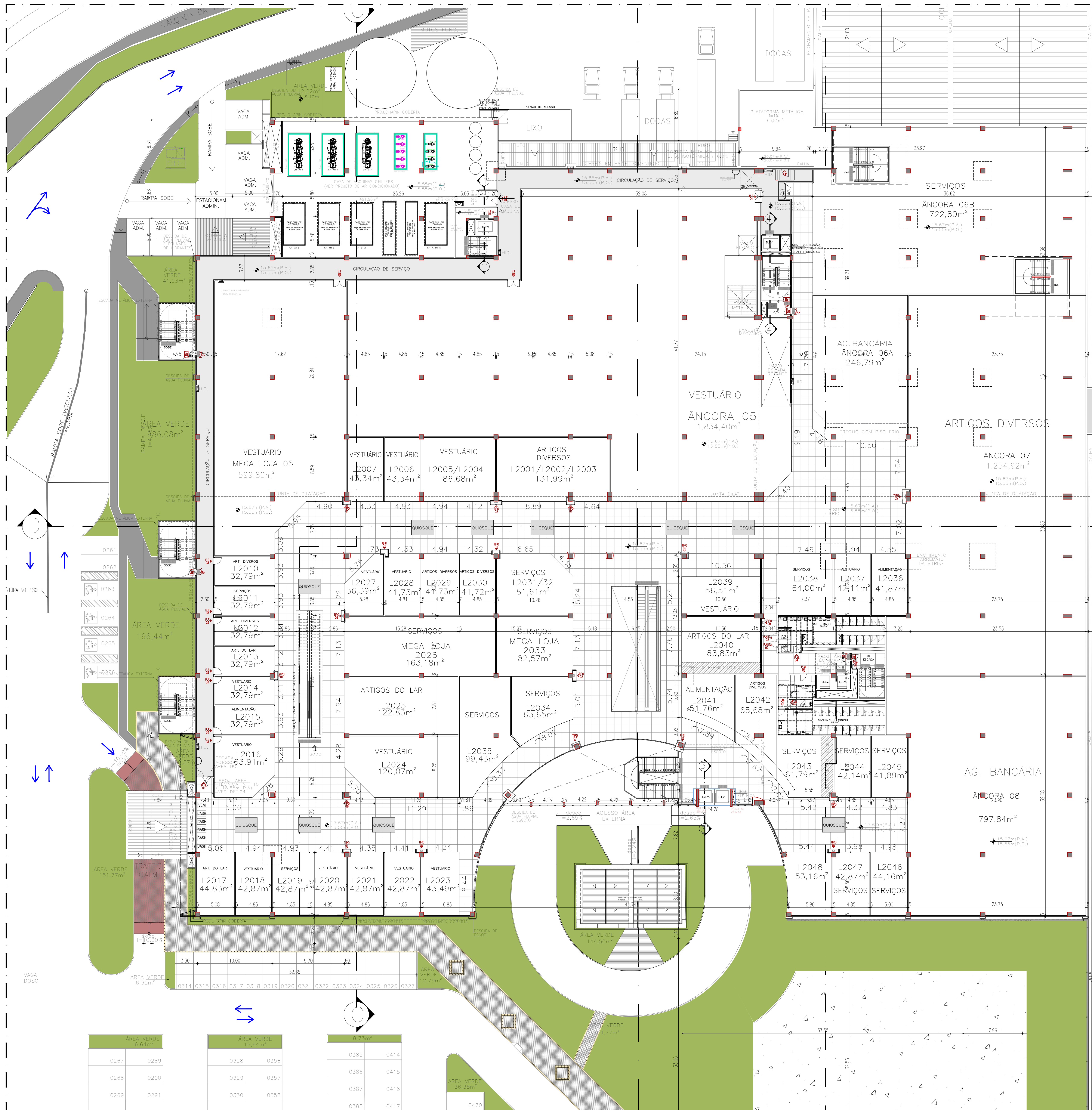
DETALHE 01 - PLANTA BAIXA PAVIMENTO L2 ESC 1/200
