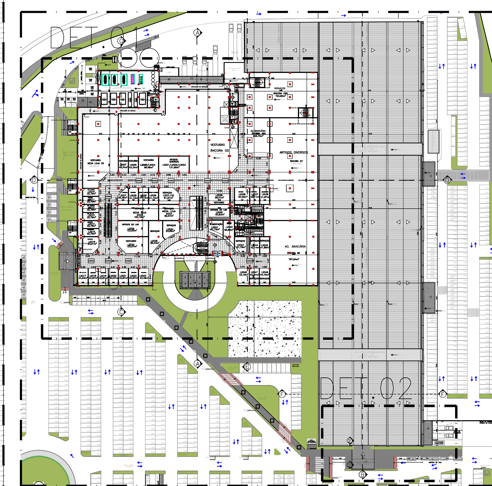
PLANTA GERAL - L2 ESC 1/1000
