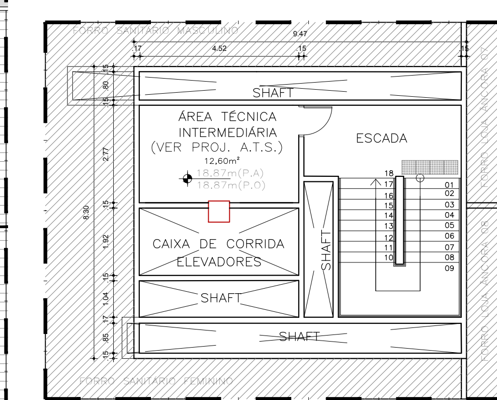
DETALHE 03 - ÁREA TÉCNICA INTERMEDIÁRIA (SANITÁRIOS) ESC 1/100
