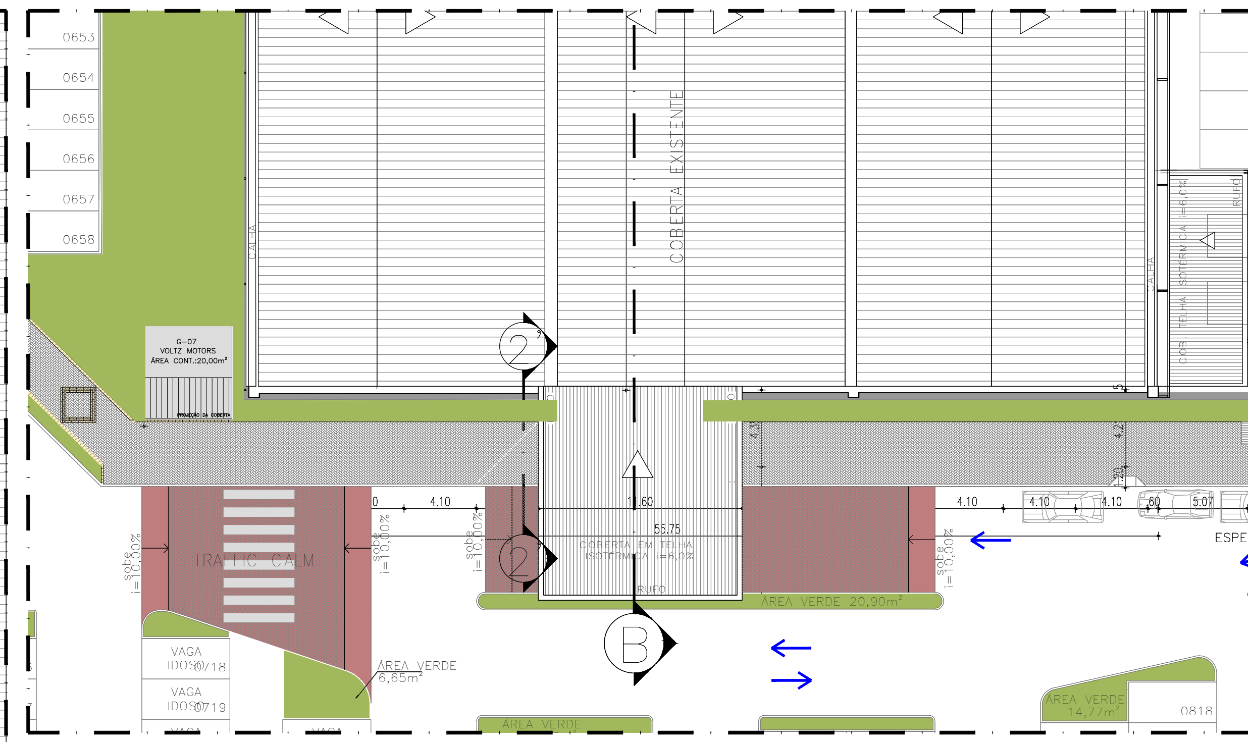
DETALHE 02 - MARQUISE ACESSO 02 GALPÃO EXISTENTE ESC 1/200
