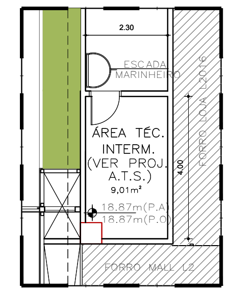
DETALHE 04 - ÁREA TÉCNICA INTERMEDIÁRIA (CIRC. SERV.) ESC 1/100
