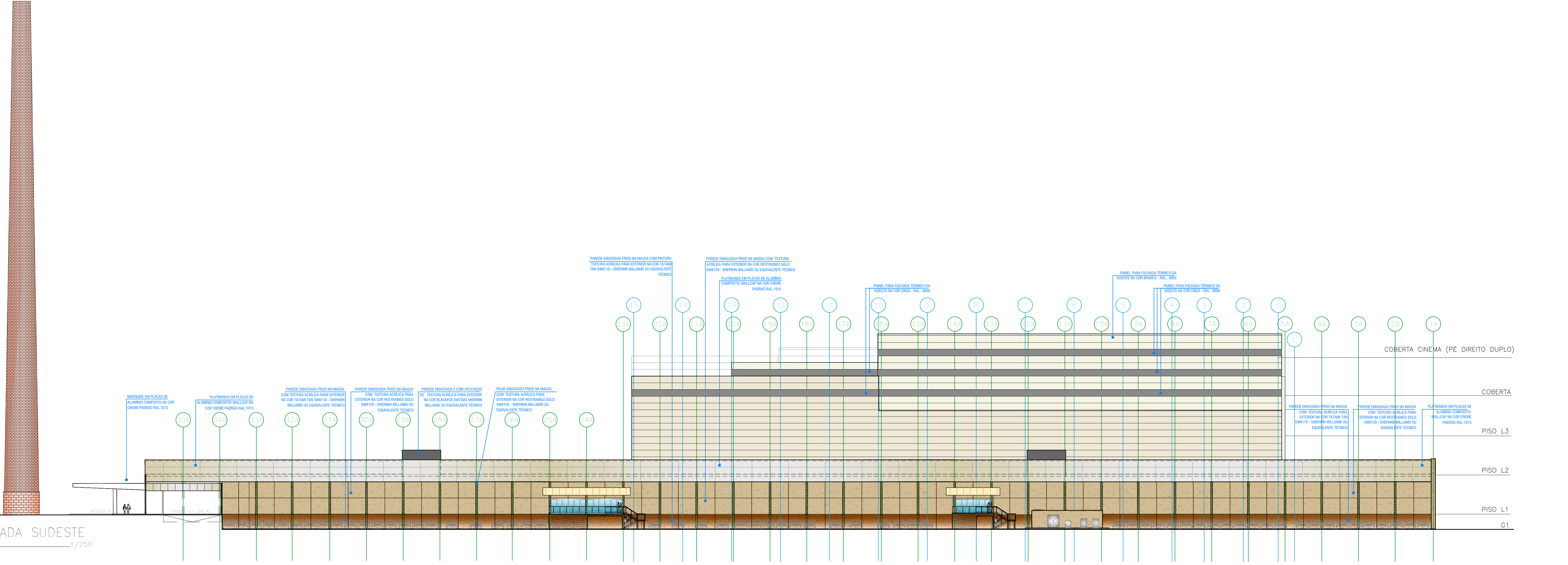
FACHADA NORDESTE ESC 1/250
